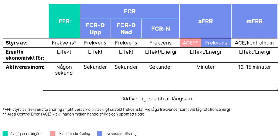
Figur 8. Stödtjänster och avhjälpande åtgärder för balansering och frekvensstabilitet. Källa: Svenska kraftnät.
