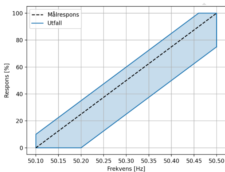
Figur 5. Delvis linjär aktivering av FCR-D ned, där Respons är andel aktiverad effekt av avropad kapacitet för FCR-D ned.
