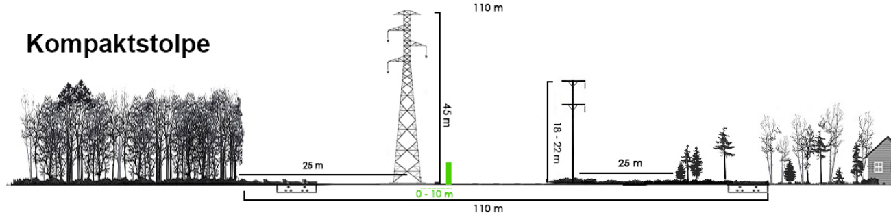
Figur 7. Illustration över ledningsgata och utredda ledningsåtgärder vid Viby, vy mot norr (bilden är inte skalenlig). Översta bilden visar exempel på nuläge med skogskant, Trafikverkets 2x65 kV, reservatsgräns (grön markering), Svenska kraftnäts 220 kV och Vattenfalls två 70 kV-ledningar. Sedan illustreras alternativ med portalstolpe där Trafikverkets ledning flyttas in i ledningsgatan och Vattenfalls ledningar kabelfieras (två alternativa placeringar utreds) och motsvarande alternativ med kombinationen tätortstolpe och kompaktjulgran. Observera att ledningsåtgärderna och placeringen är preliminära och kan komma att ändras. Den gröna markeringen motsvarar ungefärligt läge för naturreservatsgränsen och de gröna siffrorna anger ungefär hur långt in i reservatet de nya stolparna planeras.
