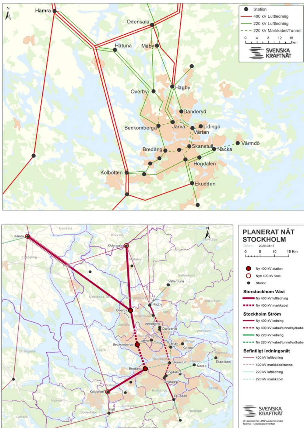
Figur 3. Schematiska bilder över Stockholms nuvarande och framtida elnät.
