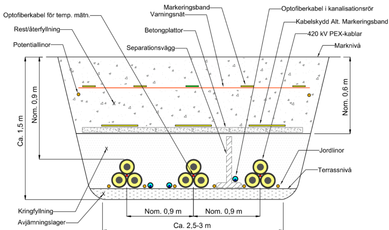
Figur 17. Preliminär pricipskiss över tvärsnitt vid en markkabelförläggning.
